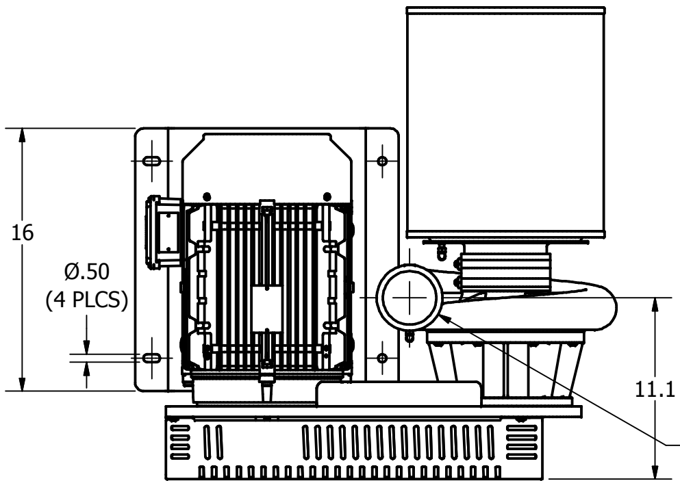
Ø4 (DISCHARGE)
